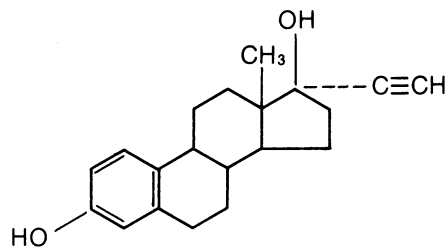
Ethinyl Estradiol C_{20}H_{24}O_2 M.W. 296.40
